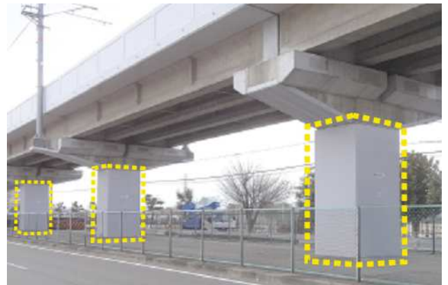
高架橋部 柱の耐震補強
